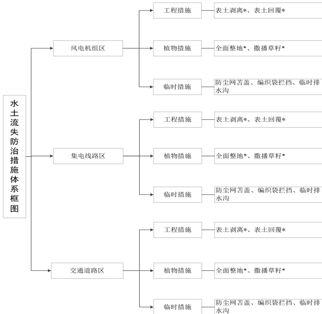
图 4.5-1 水土流失防治措施体系图 (*主体已有)
